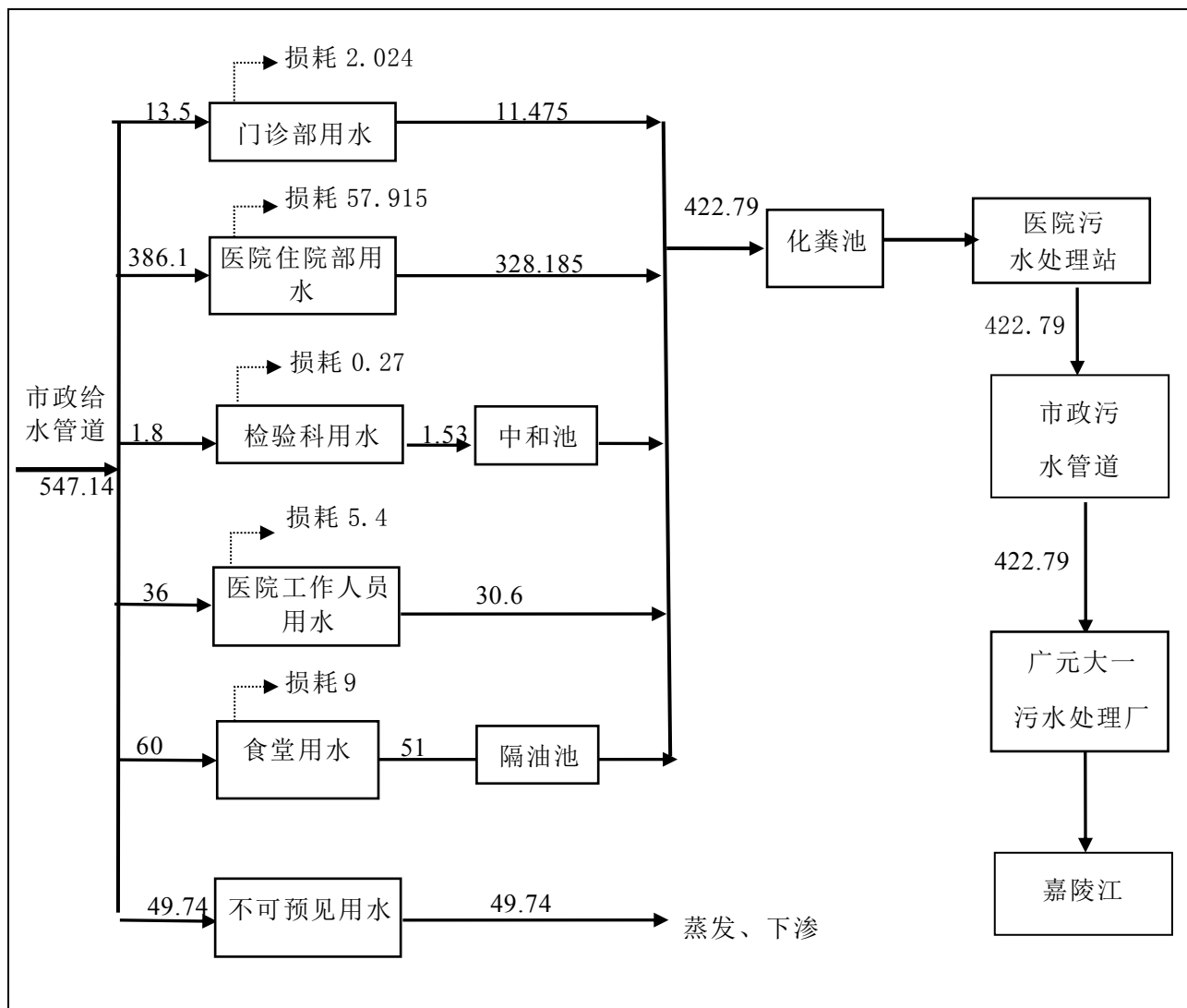
图 3.2-3 项目运营期水平衡图（单位：m 3 /d）
