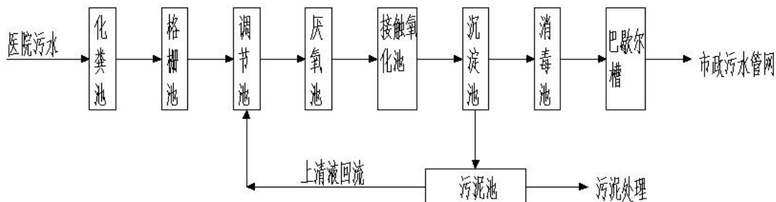
图 3.2-5 项目运营期废水处理工艺流程示意图
