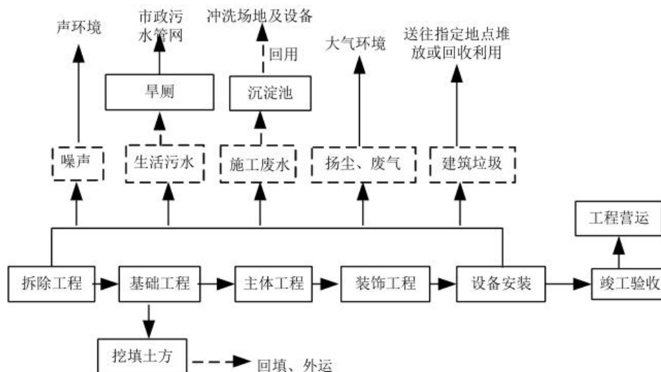
图 3.2-1 施工期工艺流程简图
