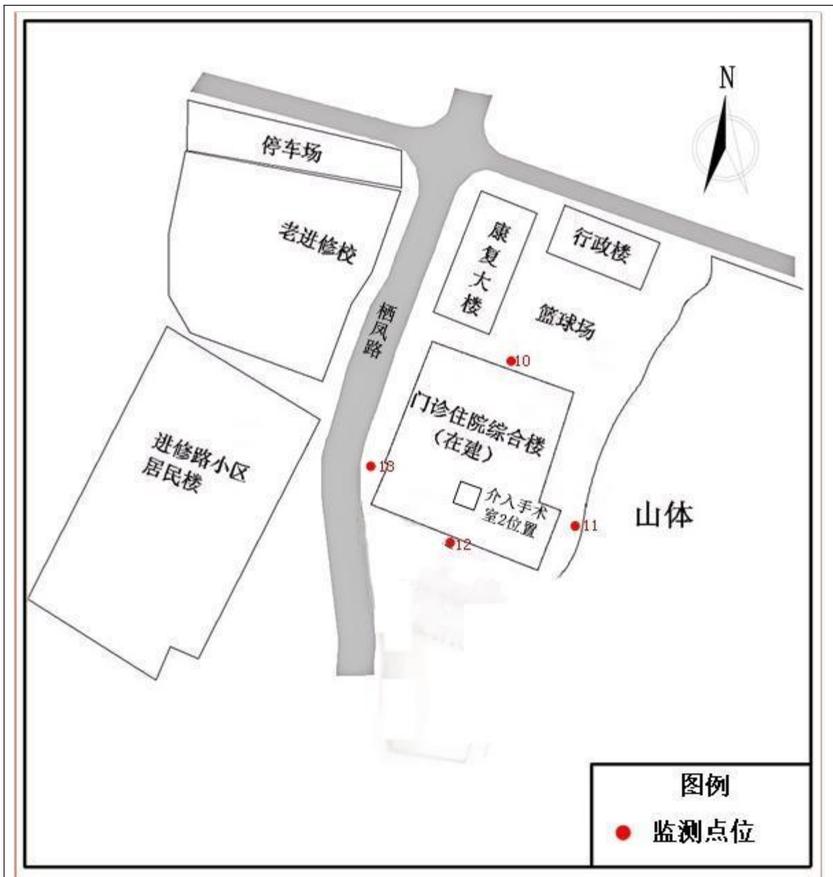
图 8-3 监测布点示意图（门诊住院综合楼外）
