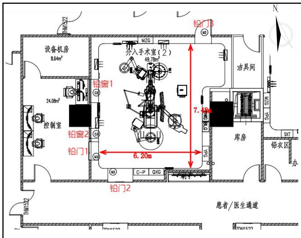
图 1-1 介入手术室 2 所在区域布局图
